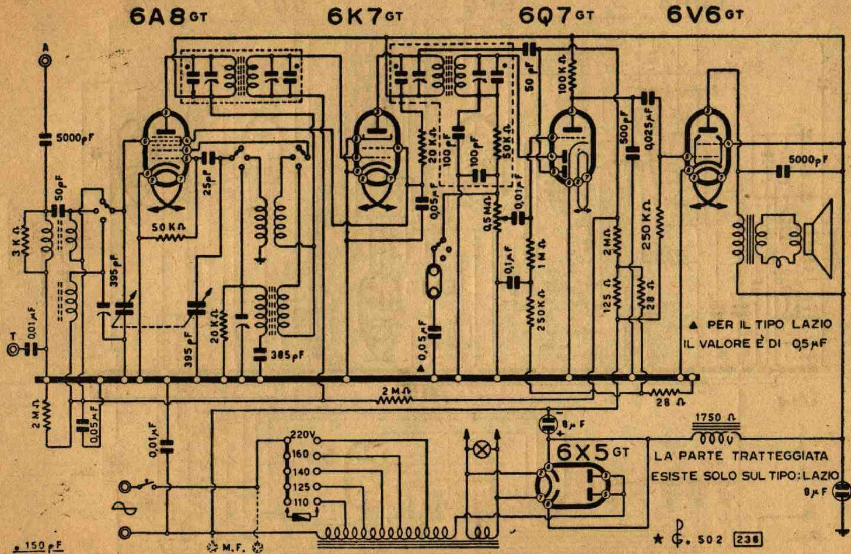
Lo schema elettrico del Sardegna e del Lazio.
